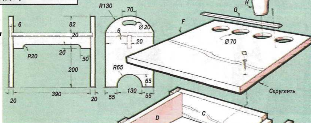
Конструкция и схема сборки столика и скамейки.
